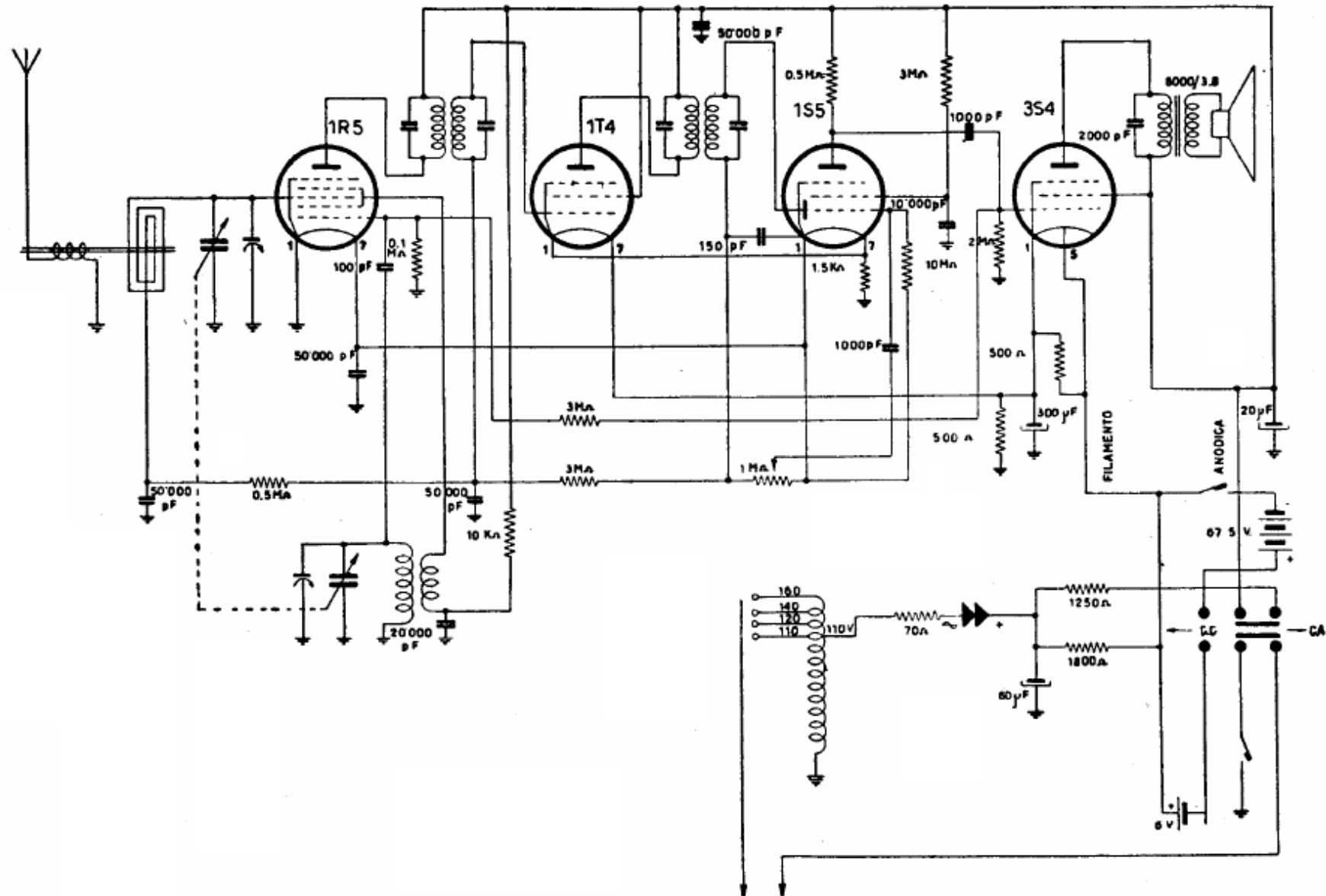
IRRADIO - Mod. BK 22 A - Apparechio portatile alimentabile con pile o con tensione alternata della rete-luce. Media frequenza 467 kc.
